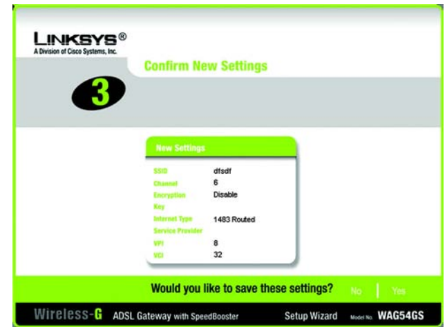
Figure 5-31 : Ecran Confirm New Settings (Confirmer les nouveaux paramètres) de l'Assistant de configuration
